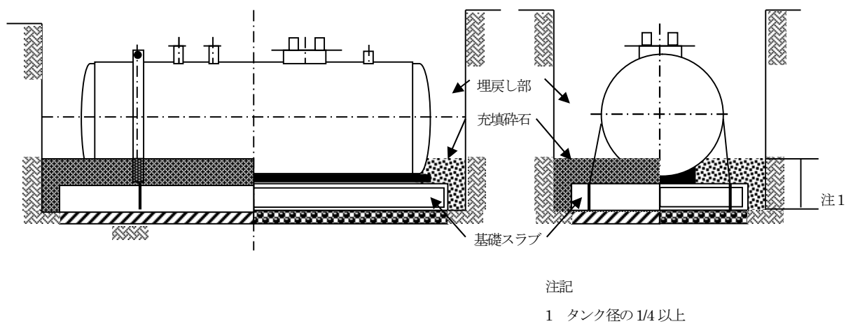
図3-2 充填碎石施工図
