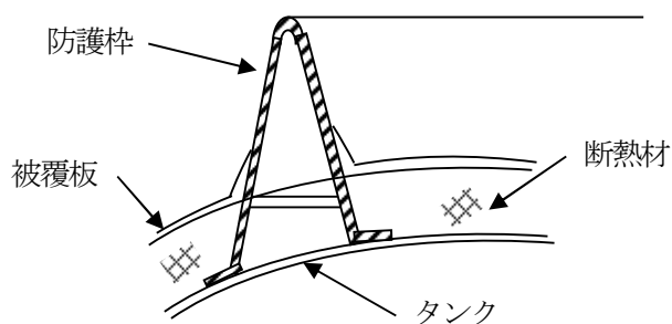
図2-8-6 タンク胴板に直接取り付ける防護枠
