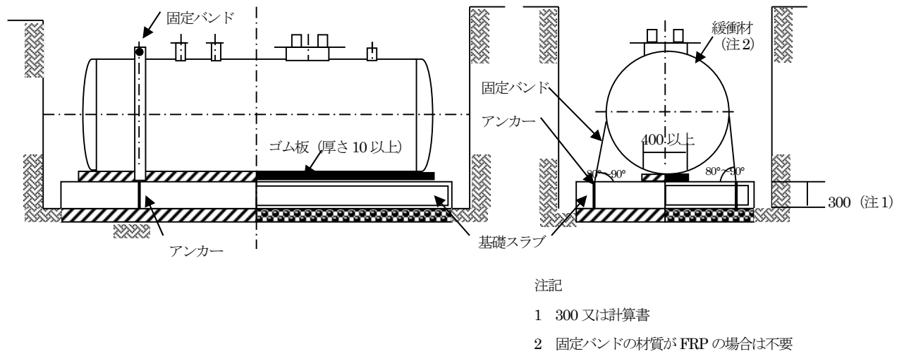
図2-1 ゴム板施工図
