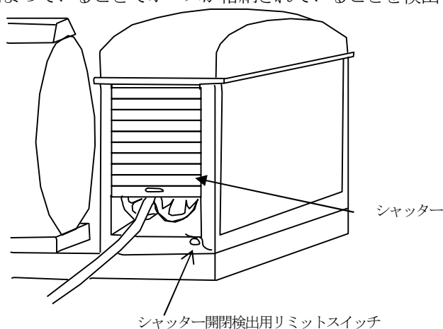
図4-2-3 給油設備の扉による方法
