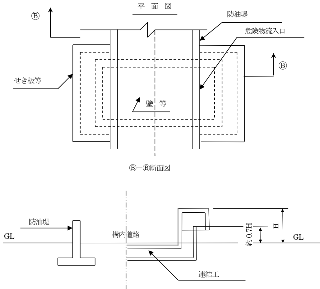
図 13-1 連結工の構造例
