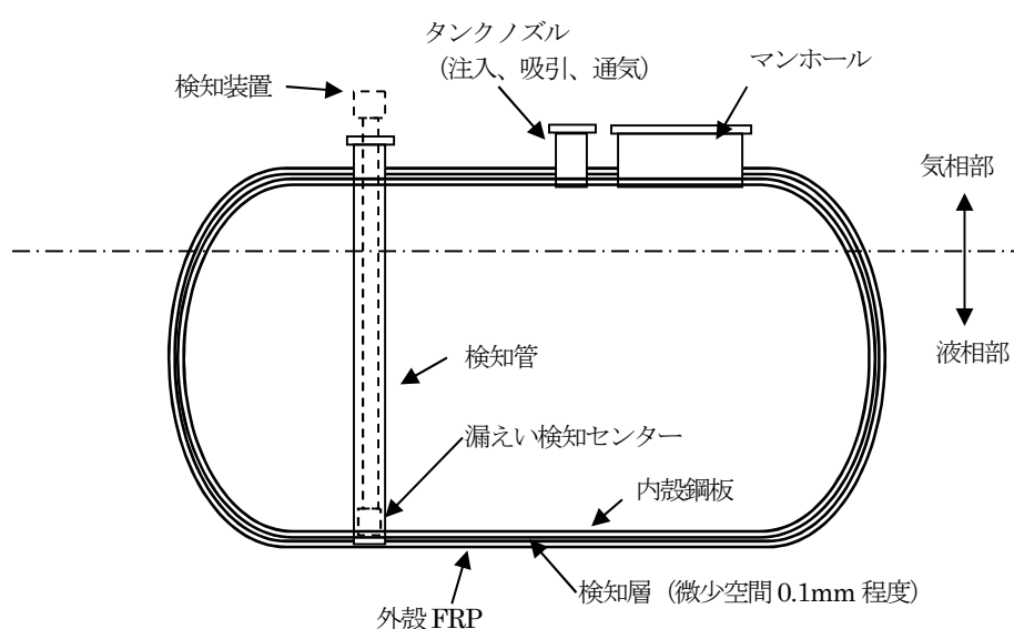
別図 - 1 構造例
