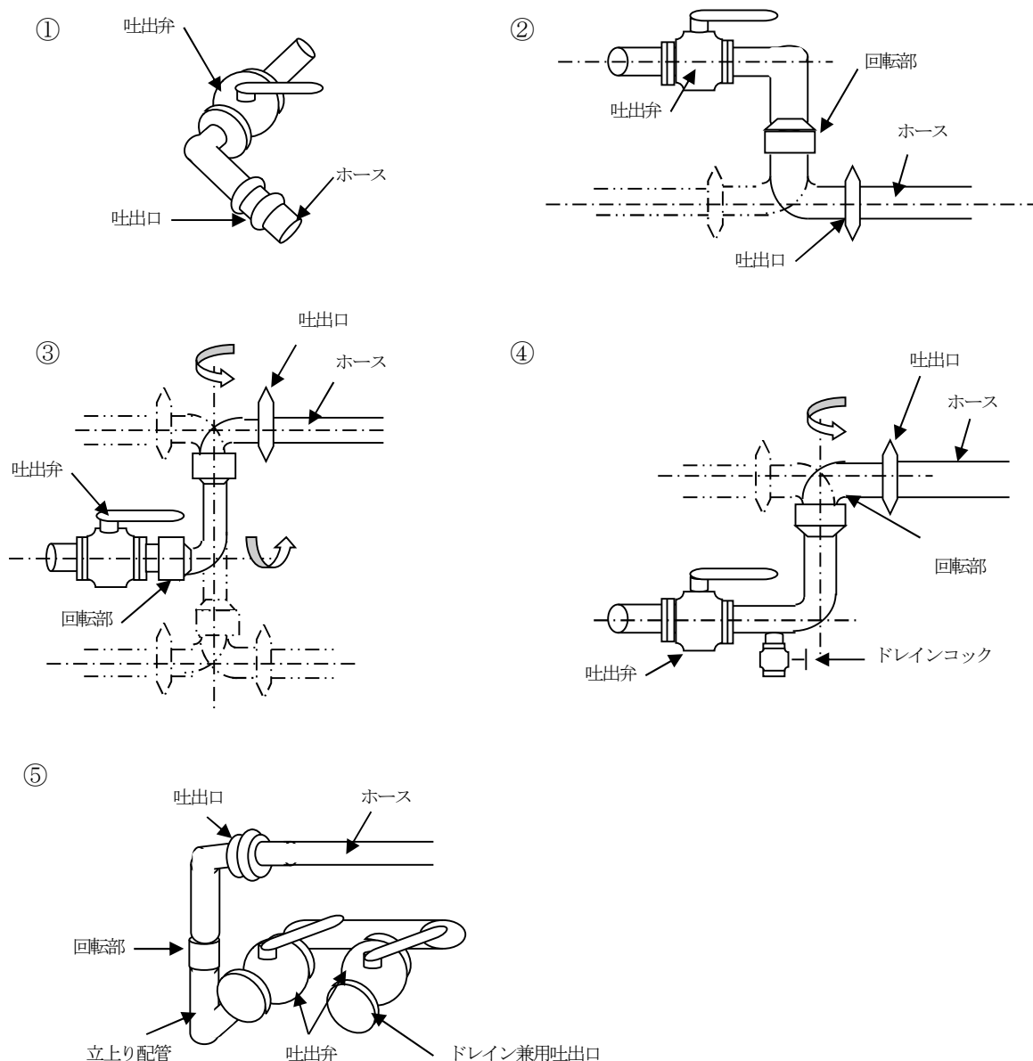
図2-14-2 配管先端部の構造
