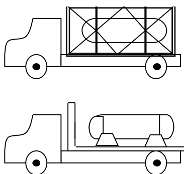
図 1-2 単一車形式で積載式の移動タンク貯蔵所の例
